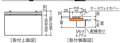
[取付上面図]
