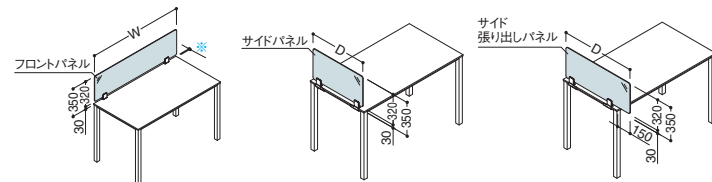
フロントパネル
