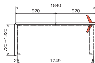
例: H1400パネルでW1800デスクをL字で囲む場合
