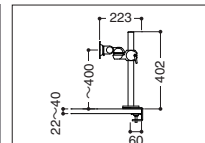
モニターアーム取付図
