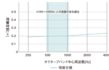
BizBreakペンタゴンタイプ吸音性能 実験結果
